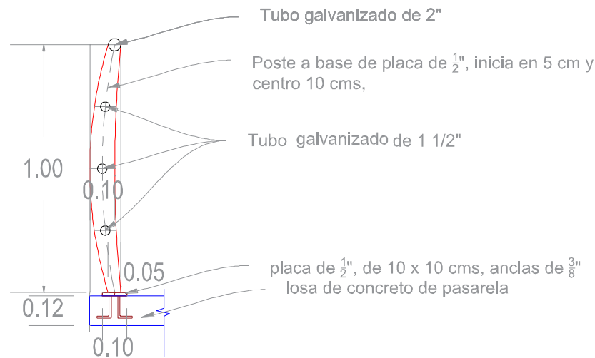
Fig. 1 Barandal de pasarela
